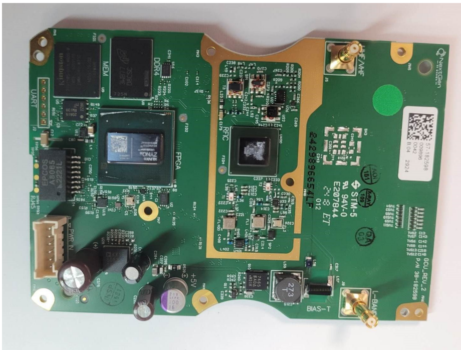
408060A Yahsat T-TAC GCU Module Bottom View
