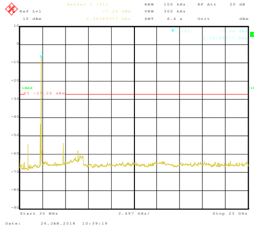
30MHz~25GHz
