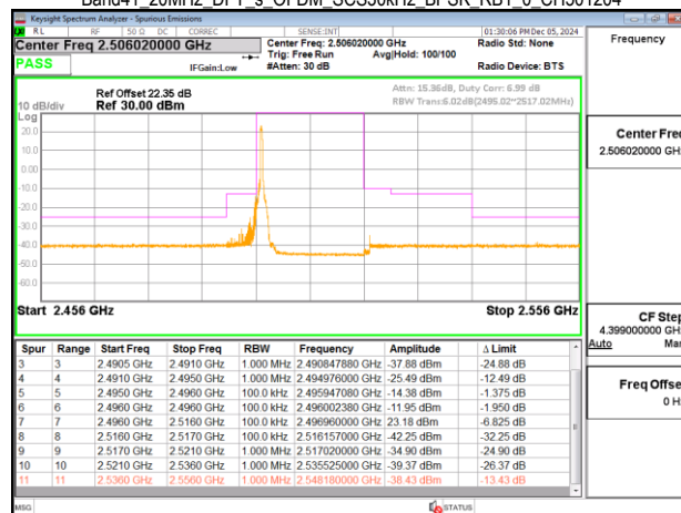
Band41_20MHz_DFT_s_OFDM_SCS30kHz_BPSK_RB1_50_CH501204
