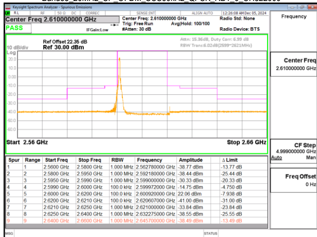
Band38_20MHz_CP_OFDM_SCS30kHz_QPSK_RB1_50_CH522000
