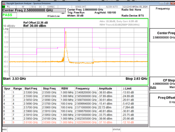
Band38_20MHz_CP_OFDM_SCS30kHz_QPSK_RB1_50_CH516000
