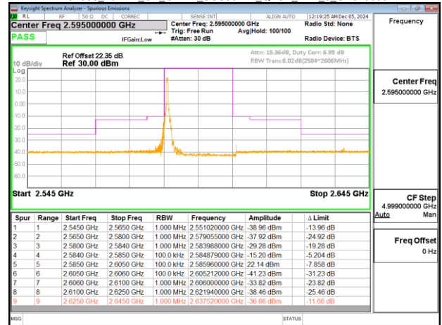
Band38_20MHz_CP_OFDM_SCS30kHz_QPSK_RB1_50_CH519000
