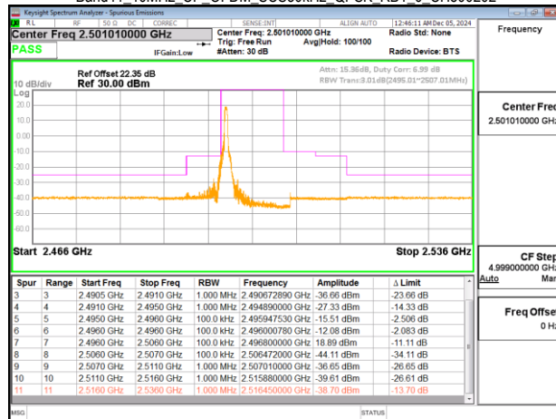
Band41_10MHz_CP_OFDM_SCS30kHz_QPSK_RB1_23_CH500202
