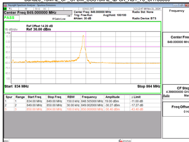
Band26_15MHz_CP_OFDM_SCS15kHz_QPSK_RB1_78_CH168300
