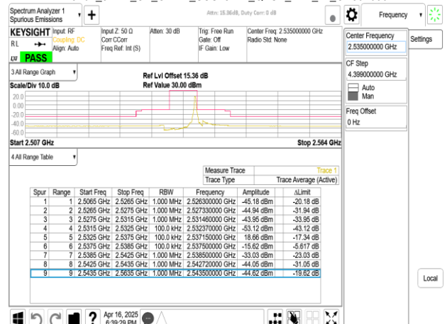
Band7_5MHz_CP_OFDM_SCS15kHz_QPSK_RB1_24_CH507000
