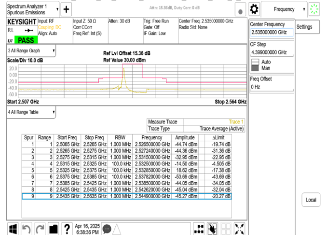
Band7_5MHz_CP_OFDM_SCS15kHz_QPSK_RB1_24_CH507000
