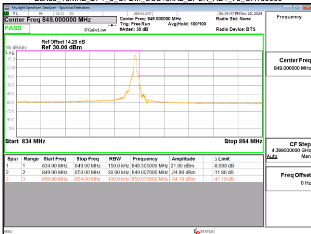
Band5_15MHz_DFT_s_OFDM_SCS15kHz_BPSK_RB1_78_CH168300
