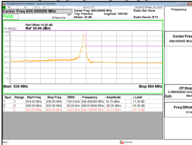
Band5_15MHz_CP_OFDM_SCS15kHz_QPSK_RB79_0_CH168300
