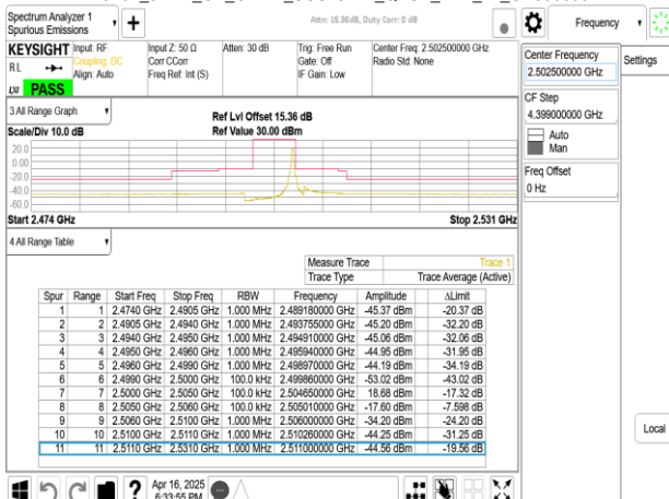
Band7_5MHz_CP_OFDM_SCS15kHz_QPSK_RB1_24_CH500500
