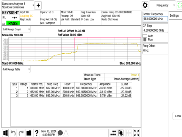
Band71_20MHz_QPSK_RB1_99_CH133372
