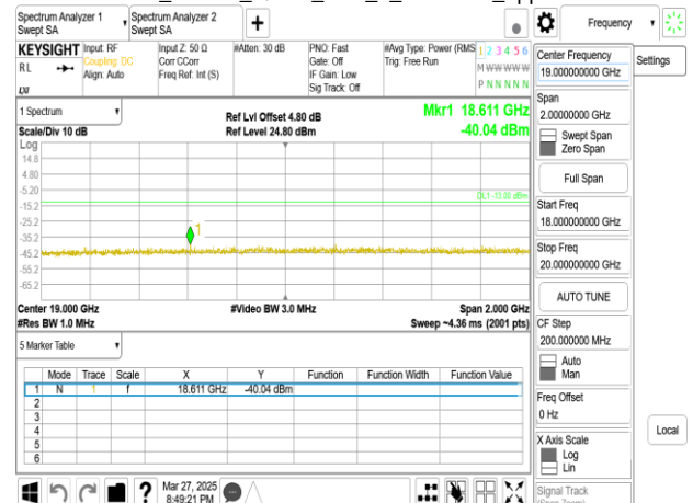
Band2_15MHz_QPSK_RB1_0_CH19125_upper 18G
