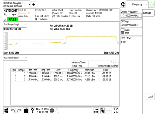
Band66_20MHz_QPSK_RB1_99_CH132572
