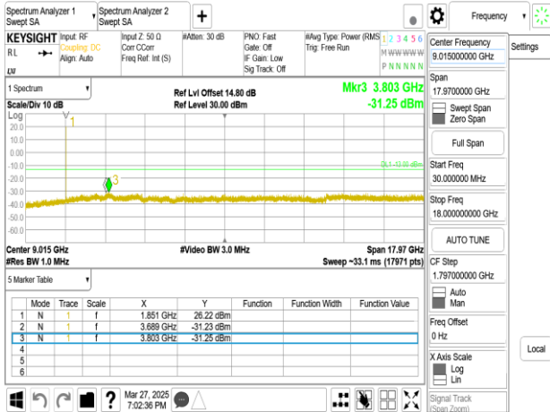
Band2_15MHz_QPSK_RB1_0_CH18675_upper 18G
