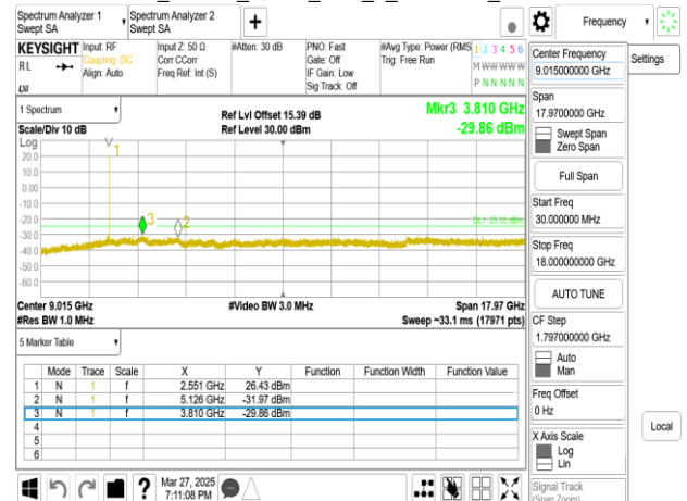
Band7_20MHz_QPSK_RB1_0_CH21350_upper 18G
