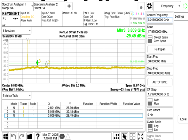
Band7_20MHz_QPSK_RB1_0_CH20850_upper 18G
