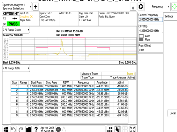
Band7_10MHz_QPSK_RB1_49_CH21400
