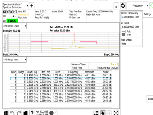
Band7_20MHz_QPSK_RB1_99_CH21100
