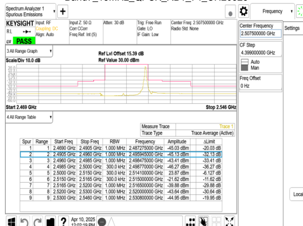
Band7_15MHz_QPSK_RB1_74_CH20825
