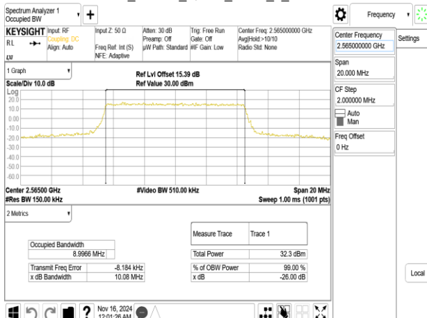
Band7_10MHz_QPSK_RB50_0_CH21400
