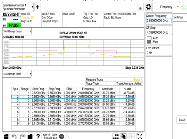
Band41_20MHz_QPSK_RB100_0_CH41490
