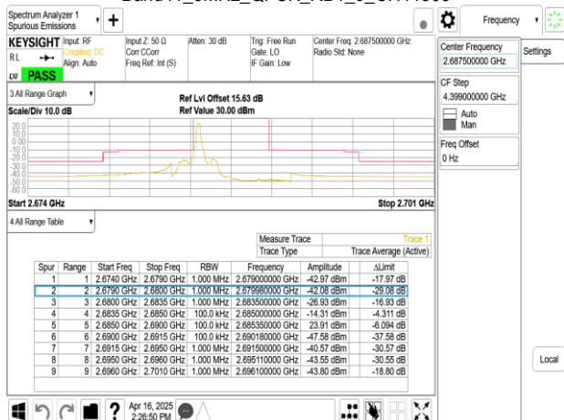
Band41_5MHz_QPSK_RB1_24_CH41565
