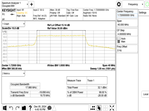
Band66_20MHz_QPSK_RB100_0_CH132072
