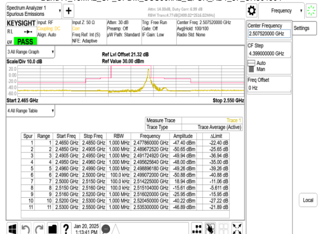
Band41_15MHz_CP_OFDM_SCS30kHz_QPSK_RB1_37_CH501504
