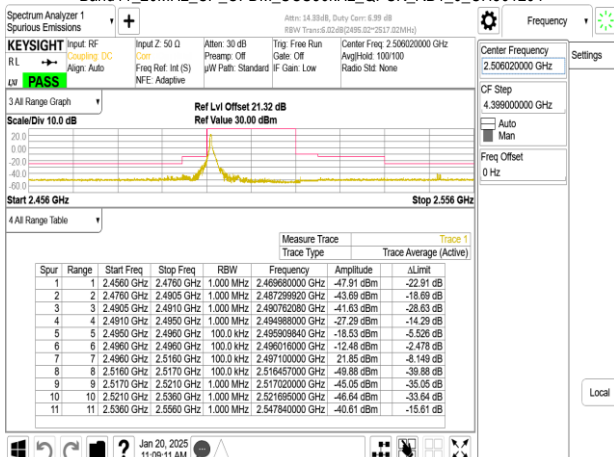
Band41_20MHz_CP_OFDM_SCS30kHz_QPSK_RB1_0_CH501204
