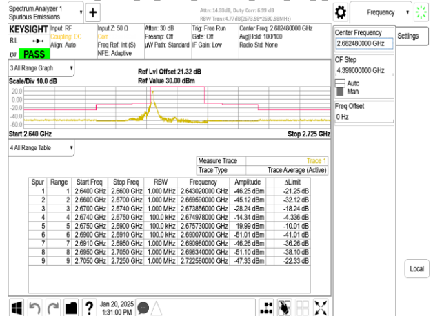
Band41_15MHz_CP_OFDM_SCS30kHz_QPSK_RB1_37_CH536496
