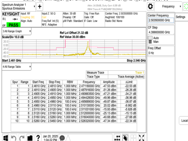
Band41_15MHz_CP_OFDM_SCS30kHz_QPSK_RB1_37_CH500700
