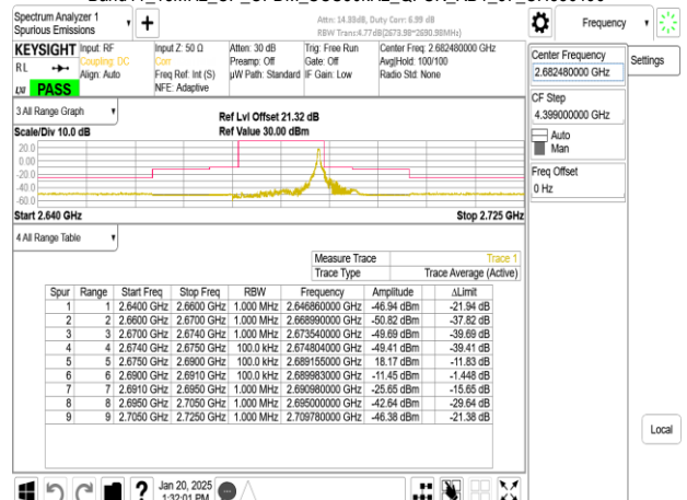
Band41_15MHz_CP_OFDM_SCS30kHz_QPSK_RB1_37_CH536496
