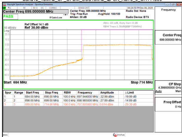
Band12_15MHz_CP_OFDM_SCS15kHz_QPSK_RB1_78_CH141700
