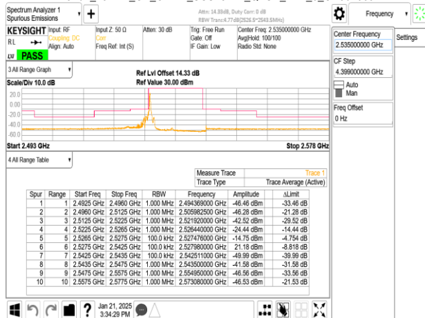
Band7_15MHz_CP_OFDM_SCS15kHz_QPSK_RB1_78_CH507000
