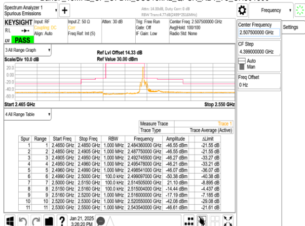
Band7_15MHz_CP_OFDM_SCS15kHz_QPSK_RB1_78_CH501500
