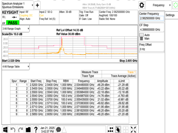
Band7_15MHz_CP_OFDM_SCS15kHz_QPSK_RB1_78_CH512500
