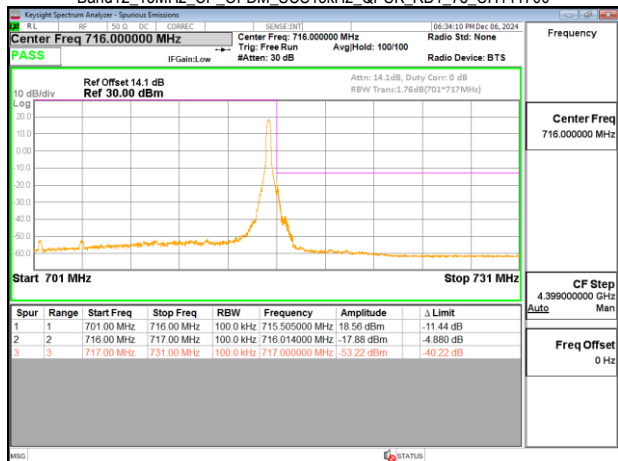
Band12_15MHz_CP_OFDM_SCS15kHz_QPSK_RB1_78_CH141700
