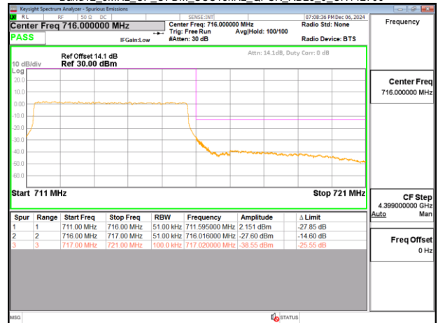
Band12 5MHz CP OFDM SCS15kHz QPSK RB25 0 CH142700
