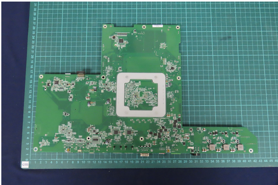
(72) EUT Photo
