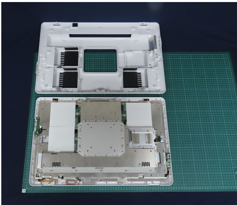
(87) EUT Photo
