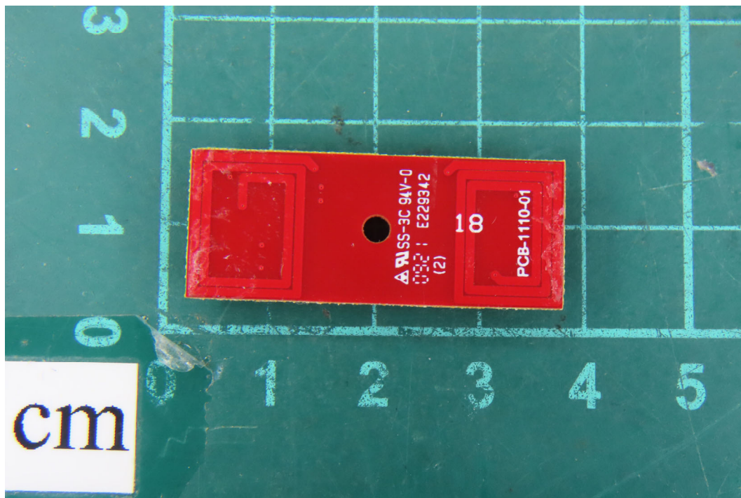
(82) EUT Photo
