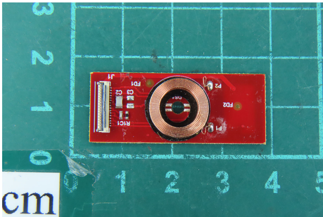
(81) EUT Photo
