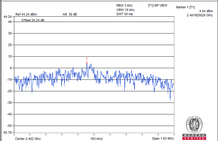
BT-LE 2M : CH 0
