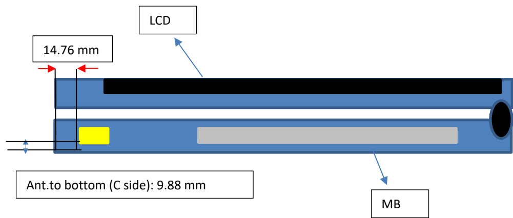
WLAN Main/Tx1
