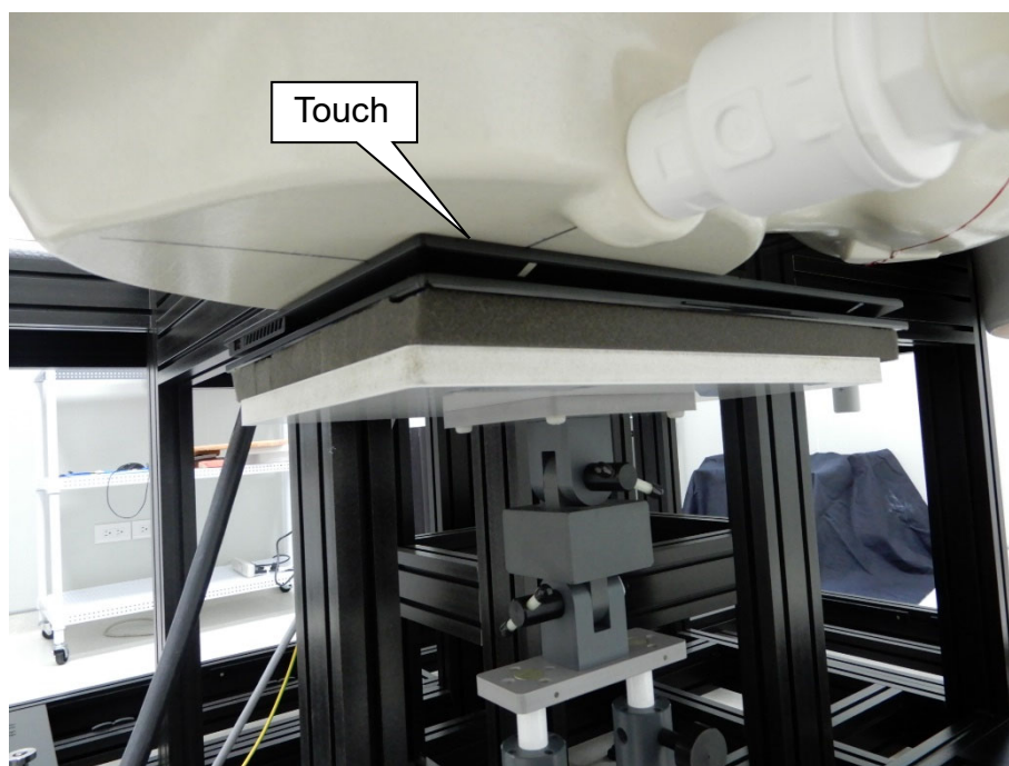
EUT Back(PAD)_Aux
