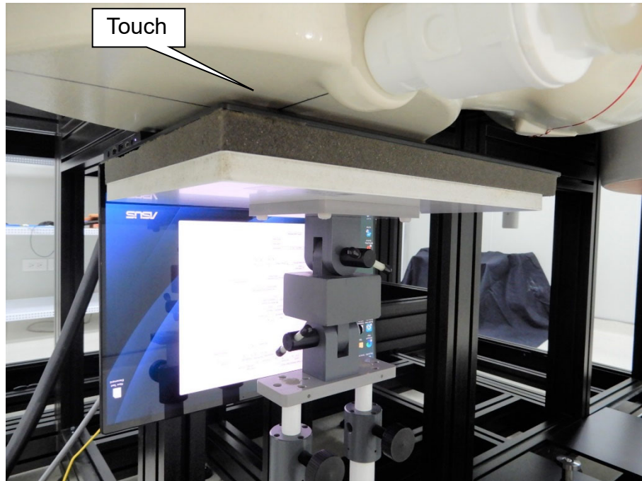
EUT Bottom(NB)_Main
