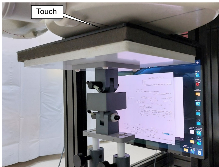
EUT Bottom(NB)_Aux
