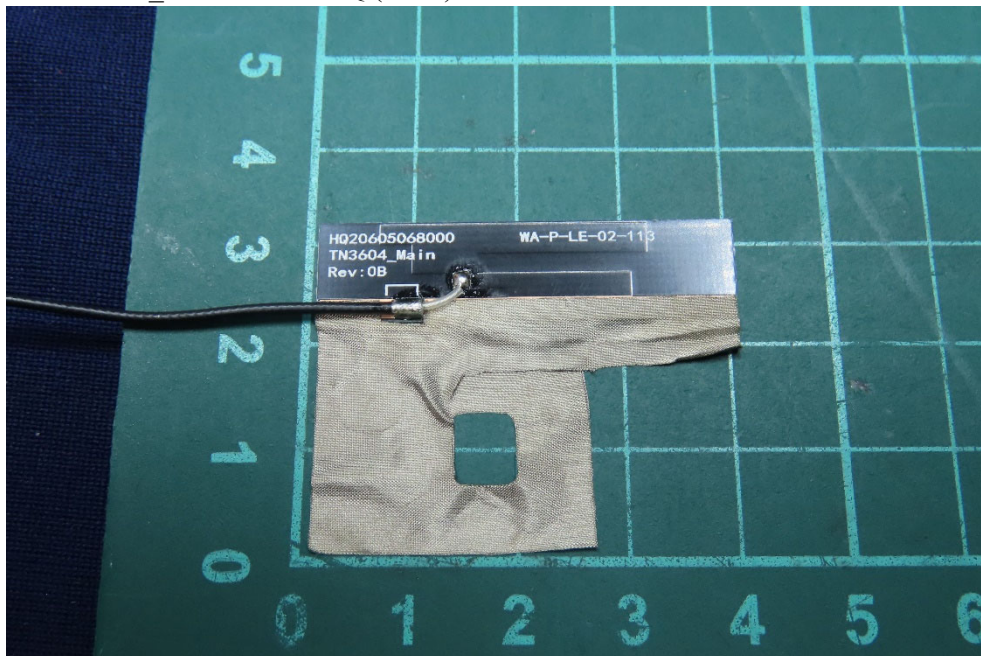
(32) EUT Photo_Antenna: INPAQ (Main)
