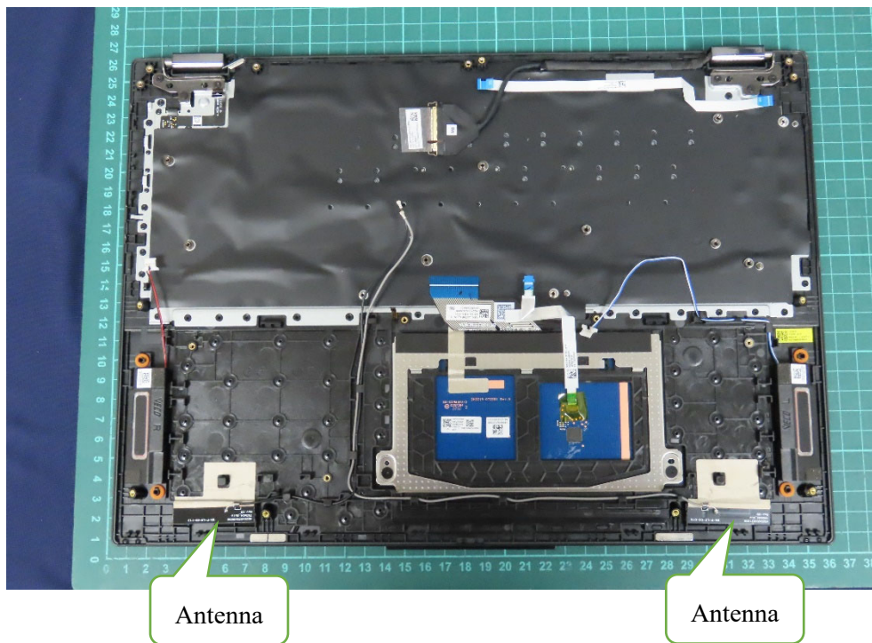
(30) EUT Photo
