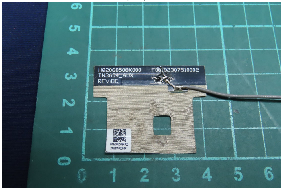
(38) EUT Photo_Antenna: INNOWAVE (Aux)
