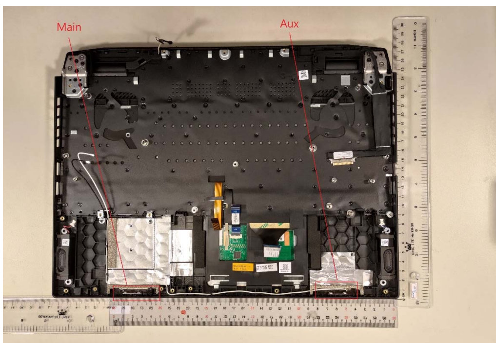
WIFI&BT Antenna
