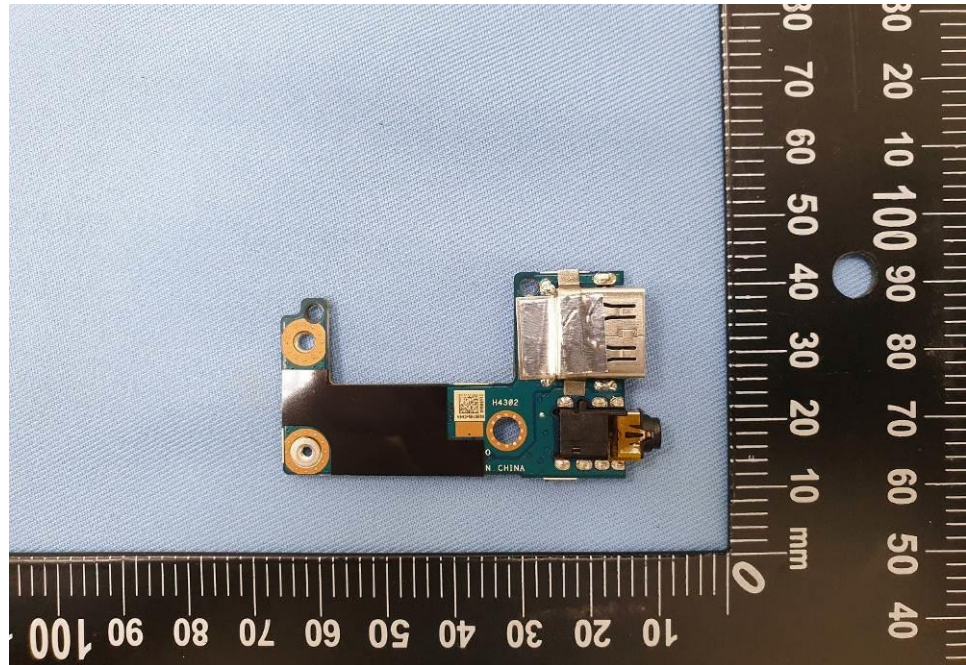
EUT Photo (17)
