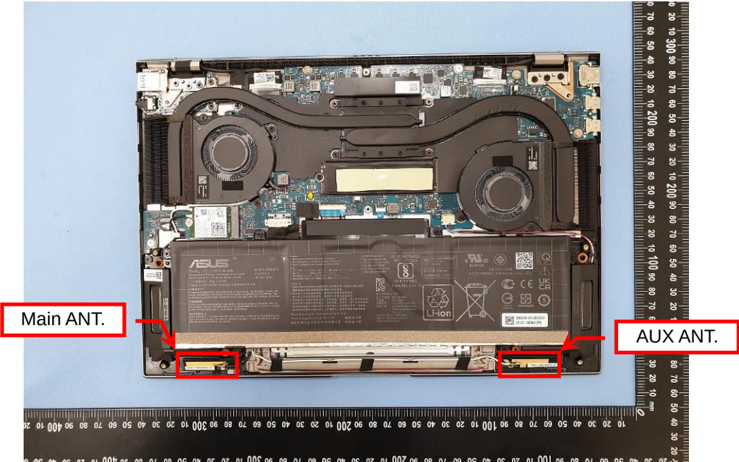
EUT Photo (2)
