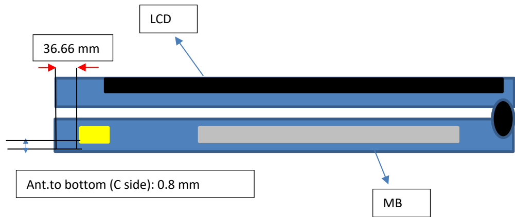
WLAN Main/Tx1
