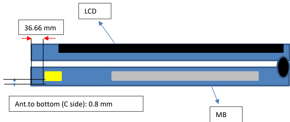
WLAN Aux/Tx2
