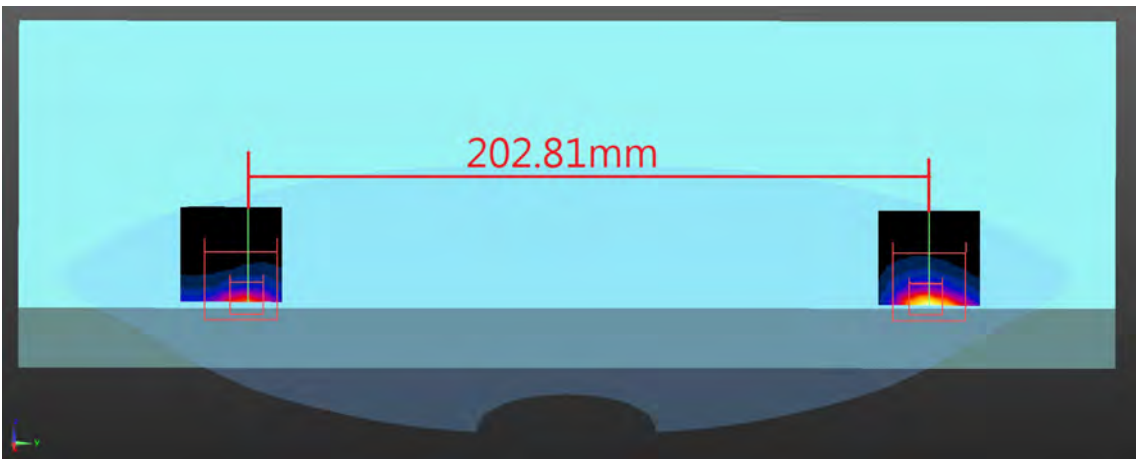
2.4G(M+BT) - Back(PAD)
