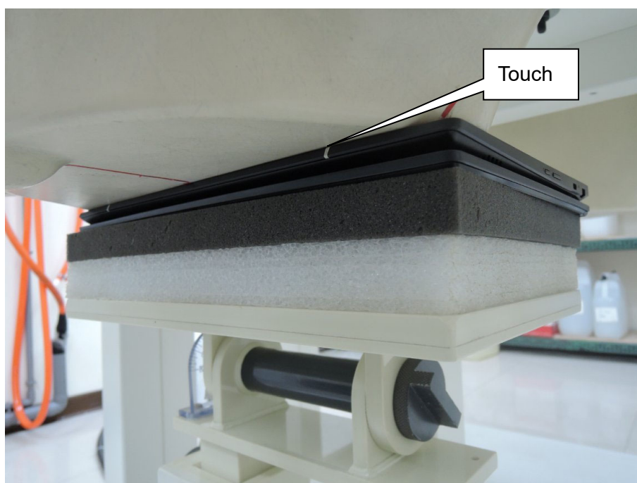
EUT Back(PAD)
