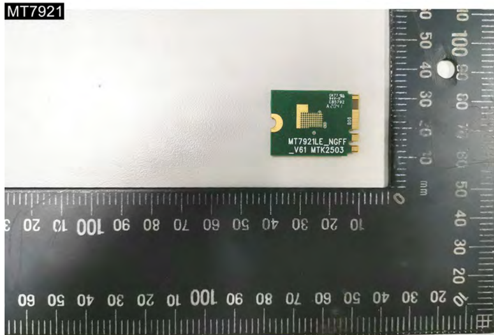
EUT Photo (4)
