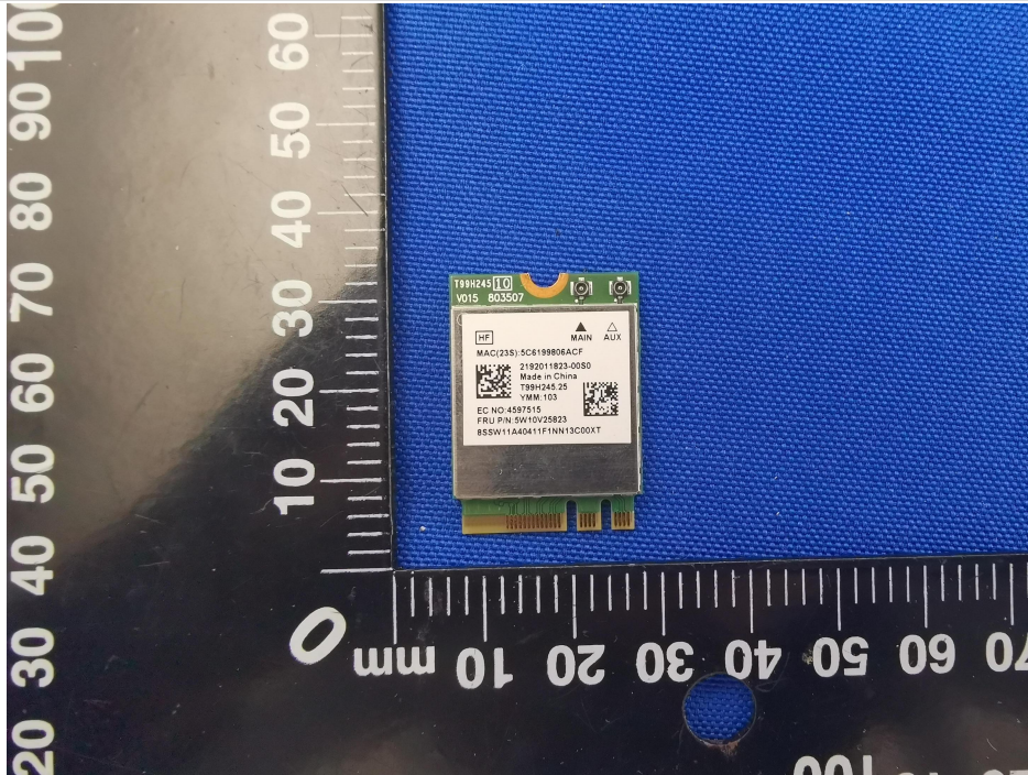
RF MODULE TOP VIEW_MT7921
