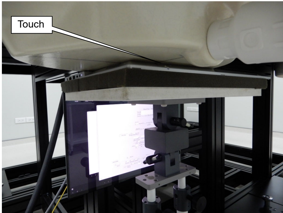
EUT Bottom(NB)_Main
