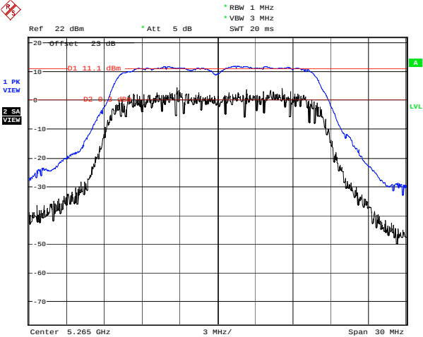
6Mb/s---5265MHz
