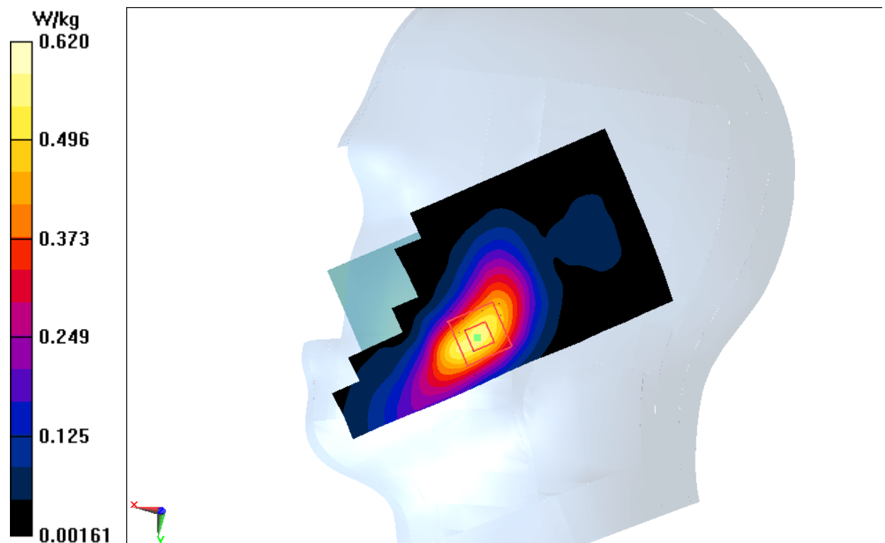
Fig.13 LTE Band7
