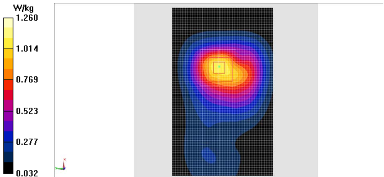
Fig.12 LTE Band4
