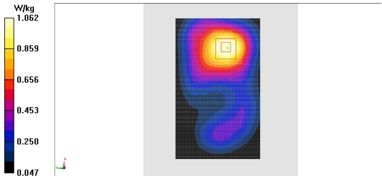
Fig.10 LTE Band2
