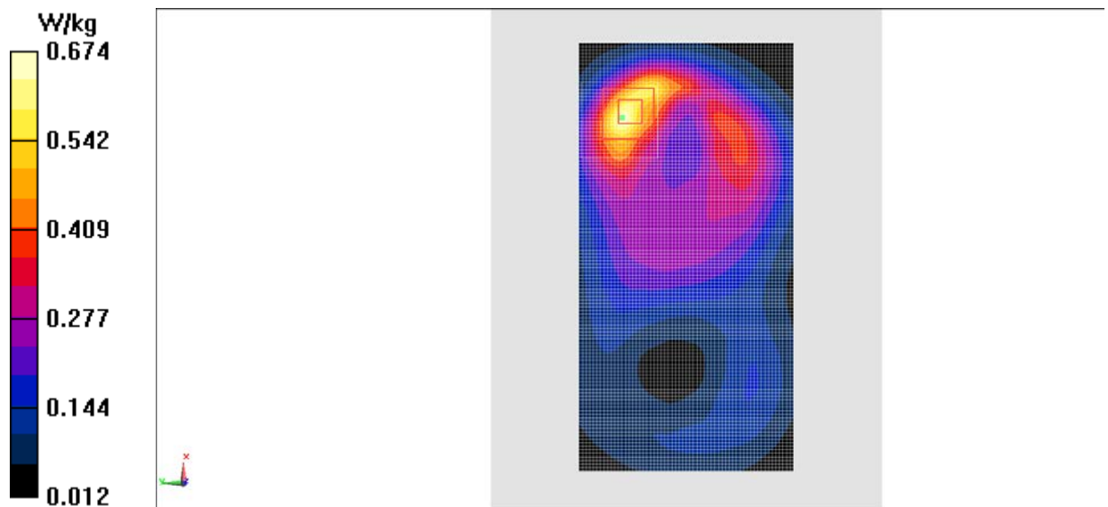
Fig.10 LTE Band2
