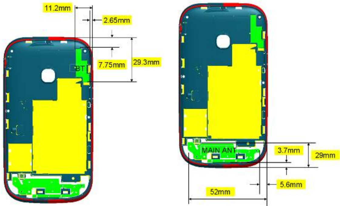
c. Antenna
