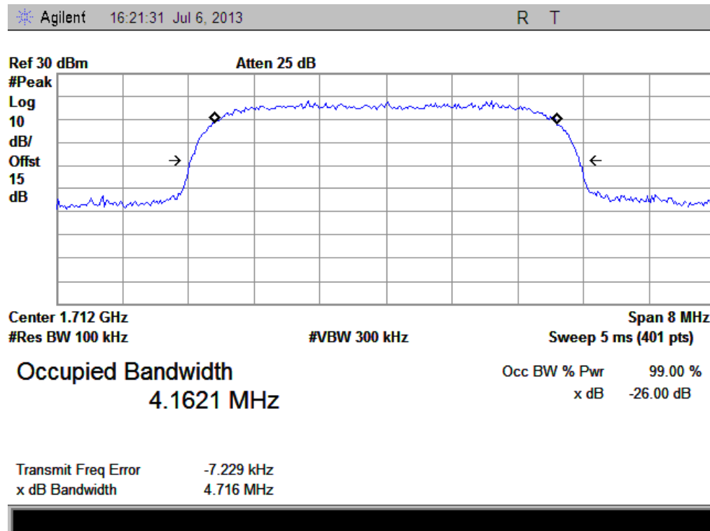
(Plot Q1: HSUPA 1700MHz Channel = 1312)
