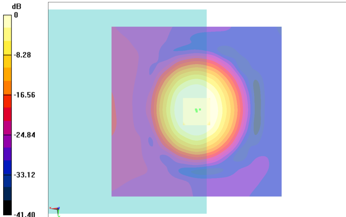
Fig B.3 T-Coil GSM 850
