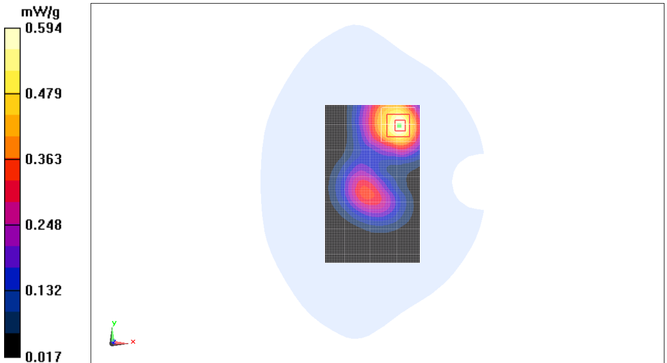
Fig. 35 1900 MHz CH810
