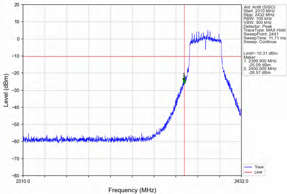
802.11n(HT20)_LCH_2412MHz_Ant8 (SISO)_NTNV
