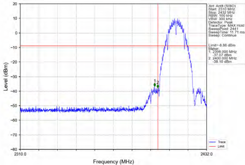
802.11b_LCH_2412MHz_Ant8 (SISO)_NTNV
