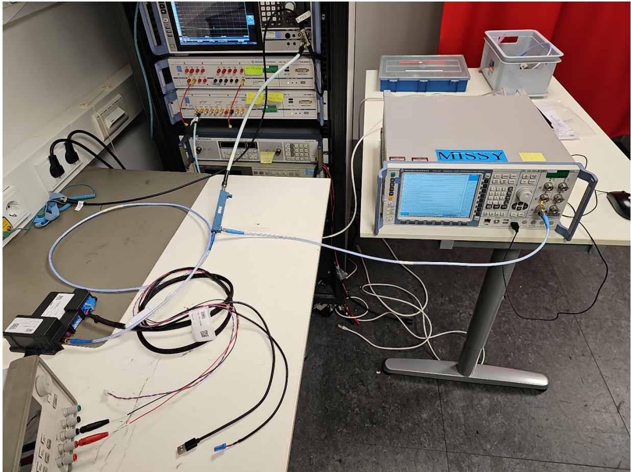
Fig. Mea.: 2 : Conducted Parameter Image 2
