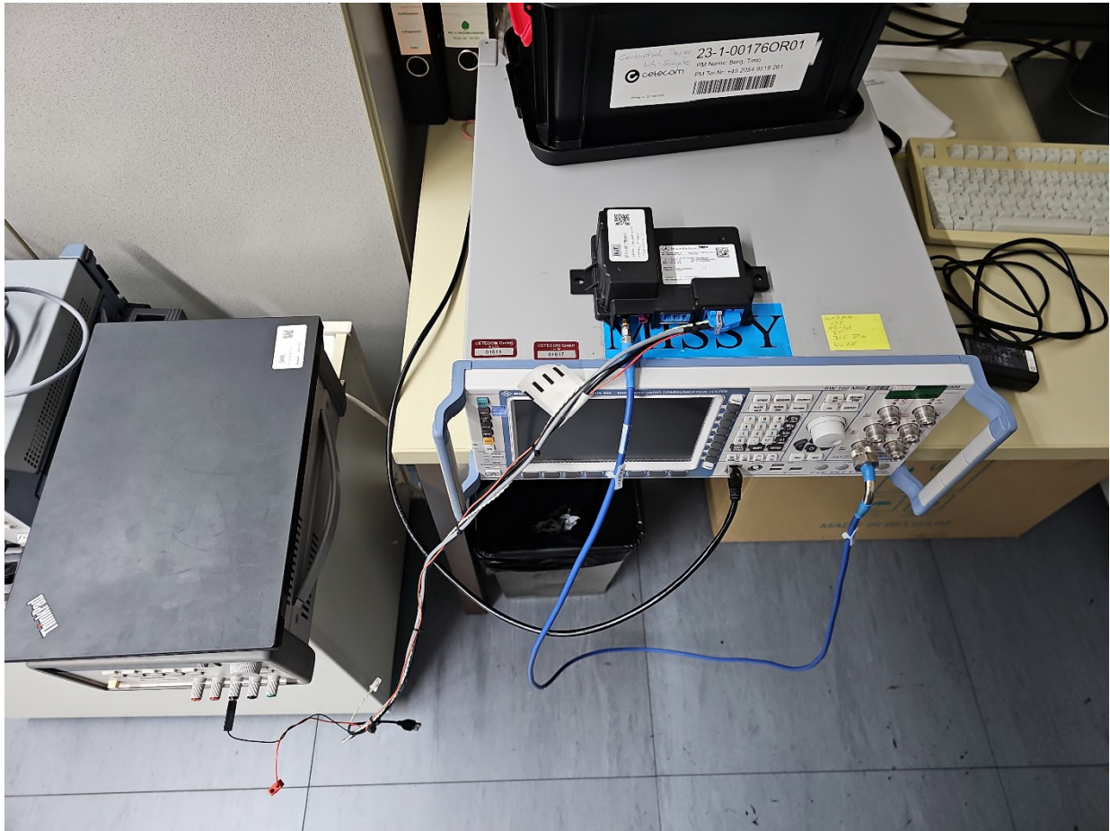
Fig. Mea.: 1 : Conducted Parameter Image 1
