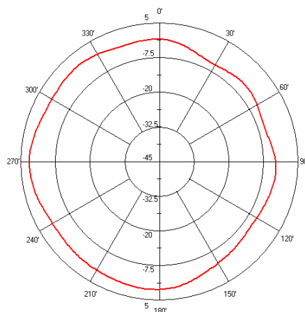
AN9520 E-Plane
