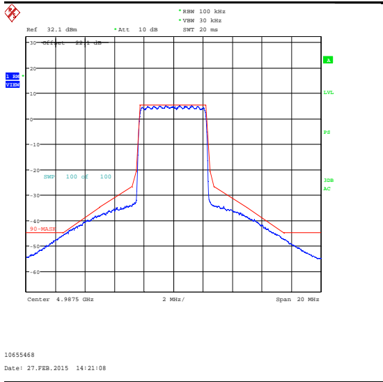
QPSK
