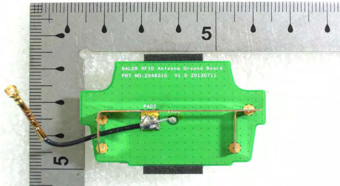
GPS Antenna
