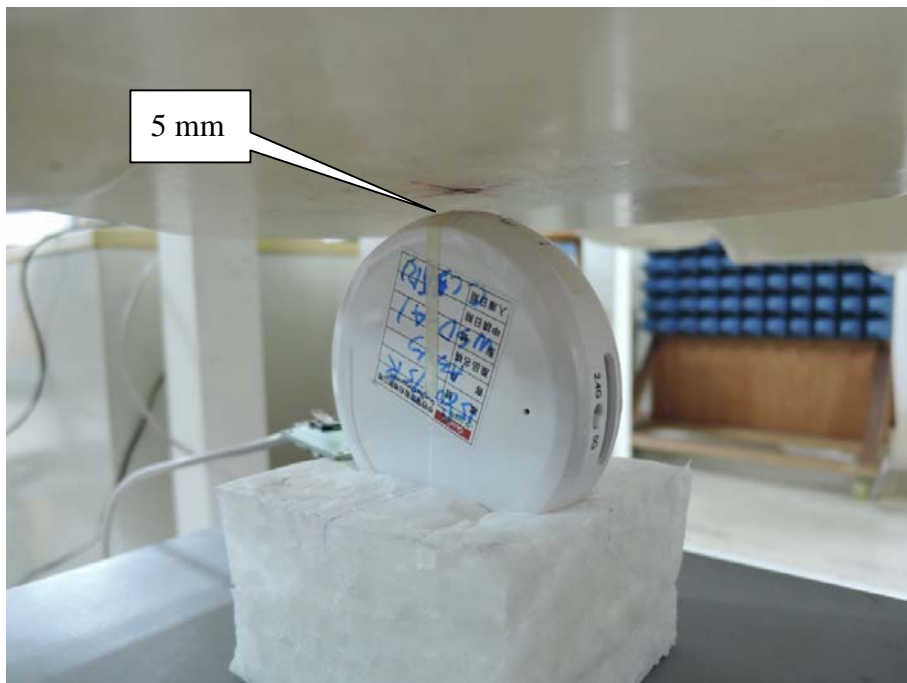
EUT Left-Side 2
