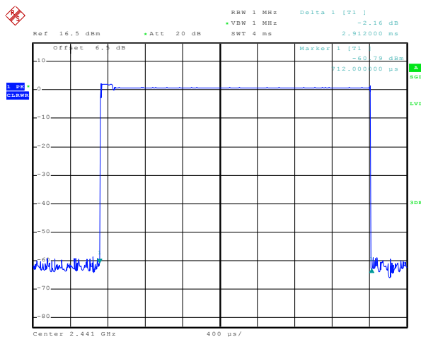
2-DH5
