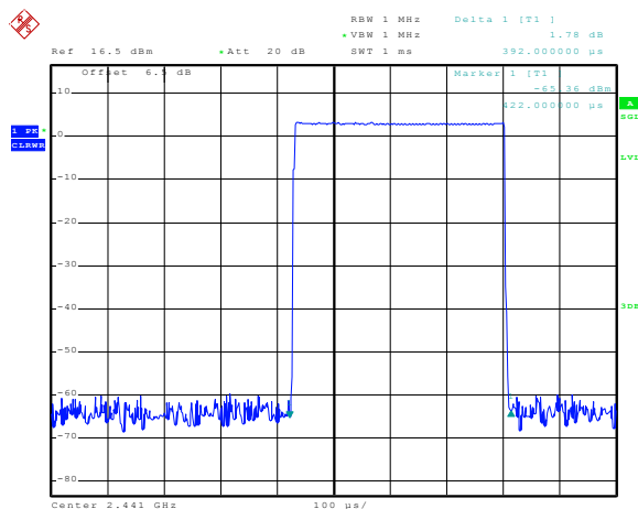
DH1
