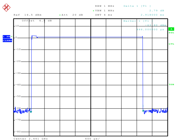
3-DH5
