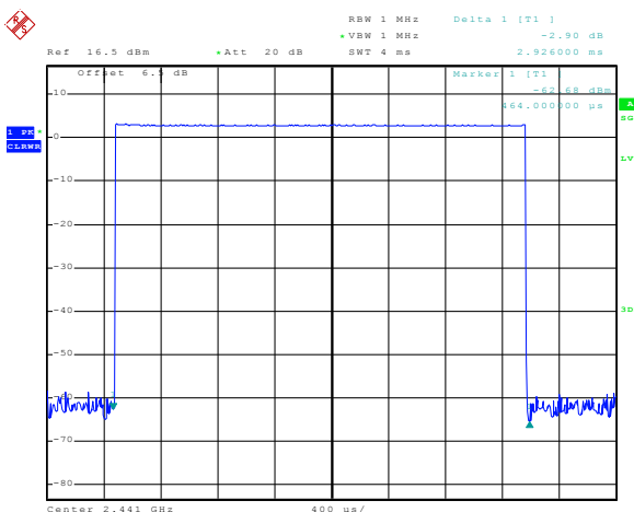
DH5
