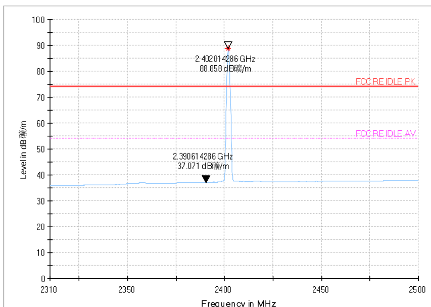
AV detector
