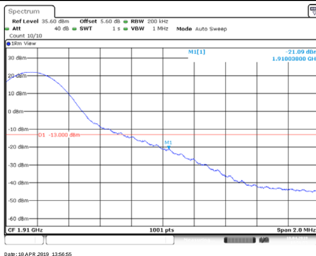
Band2 15MHz 16QAM 19125 75RB#0
