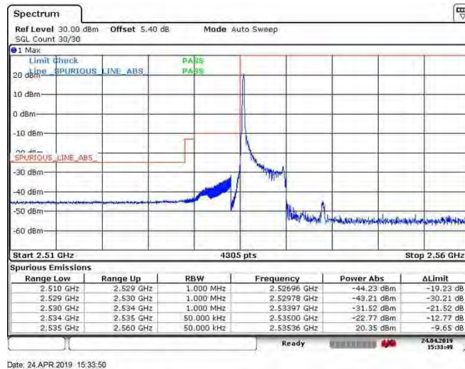
Band41_5MHz_QPSK_40065_25RB#0
