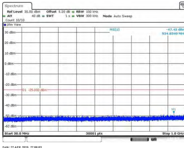
Band41_20MHz_QPSK_40640_1RB#0
