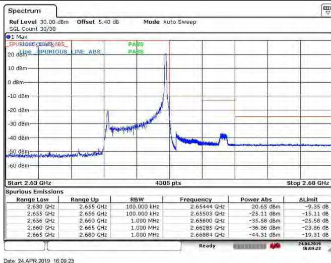
Band41_10MHz_QPSK_41190_50RB#0
