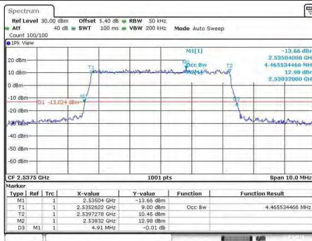
Band41_5MHz_QPSK_40065_25RB#0
