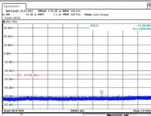
Band38_20MHz_QPSK_37850_1RB#0
