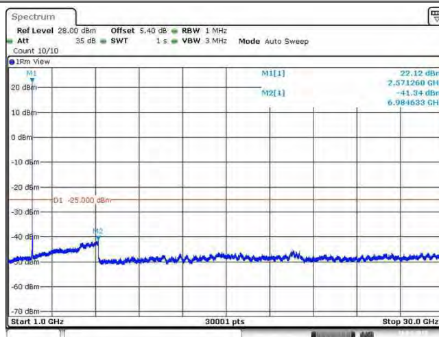
Band38_20MHz_QPSK_37850_1RB#0
