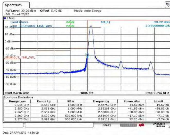
BAND38_20MHz_QPSK_37850_100RB#0
