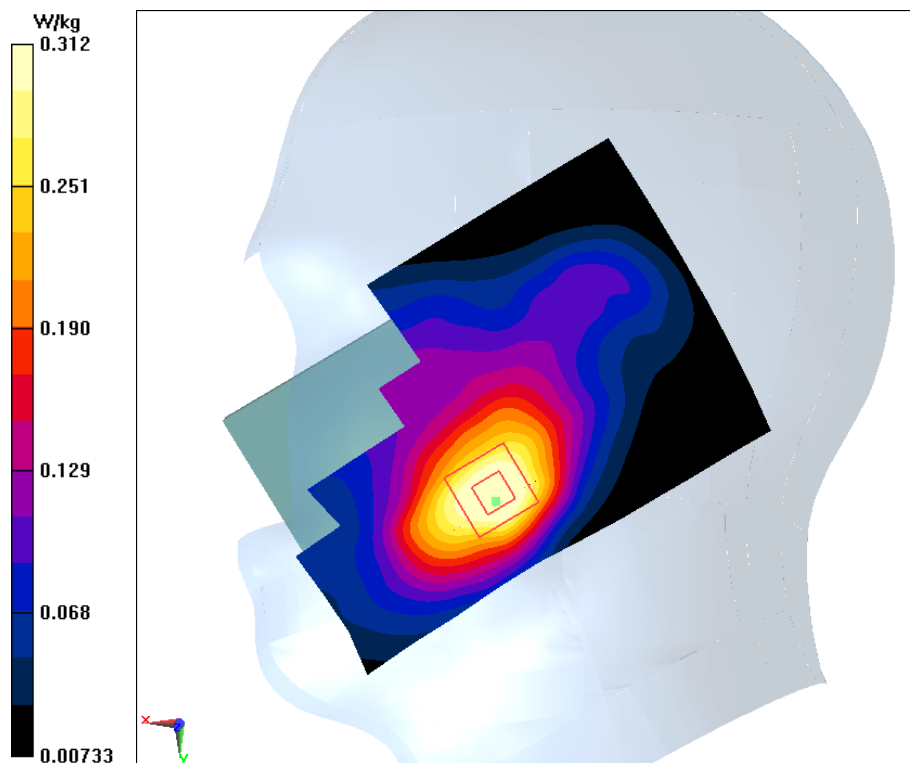
Fig.13 LTE Band4
