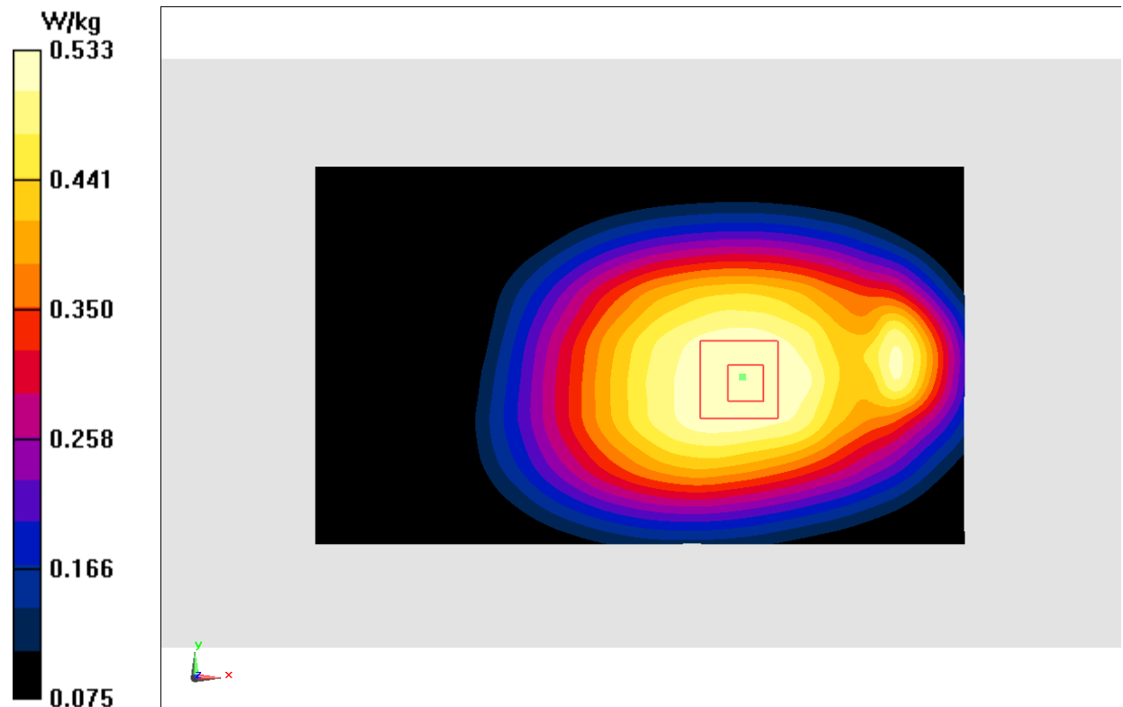
Fig.6 WCDMA 850
