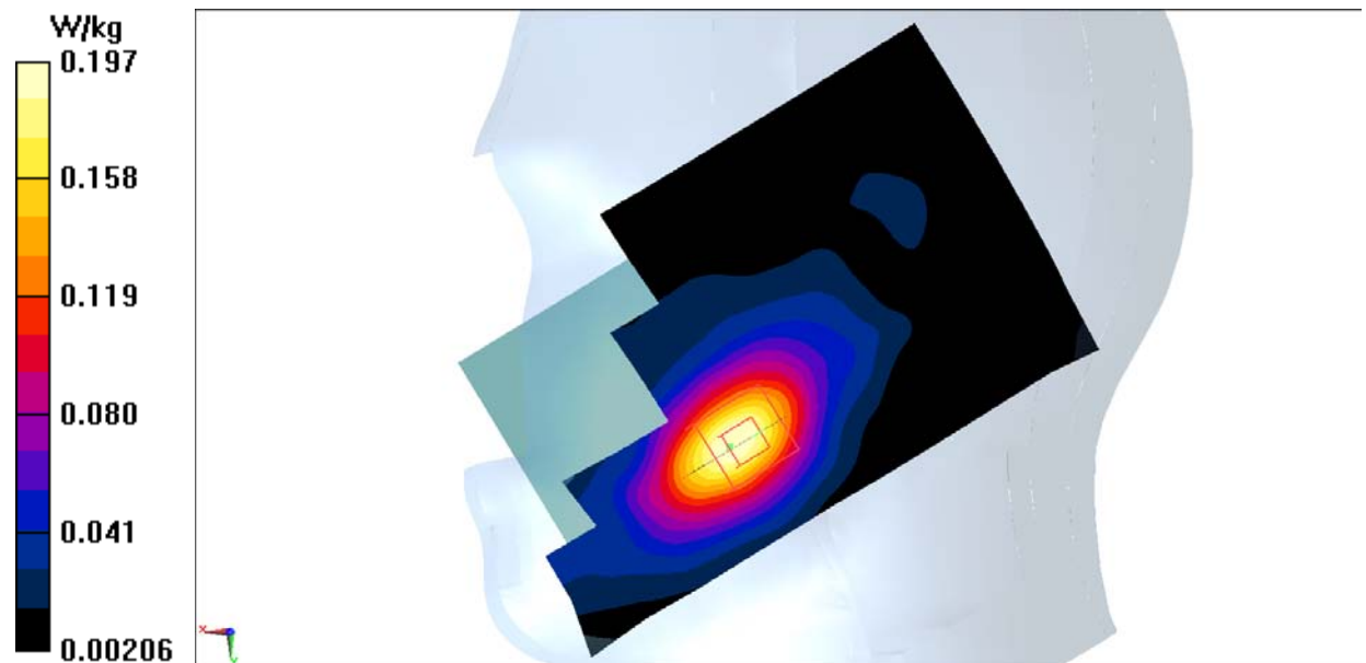
Fig.9 WCDMA1900
