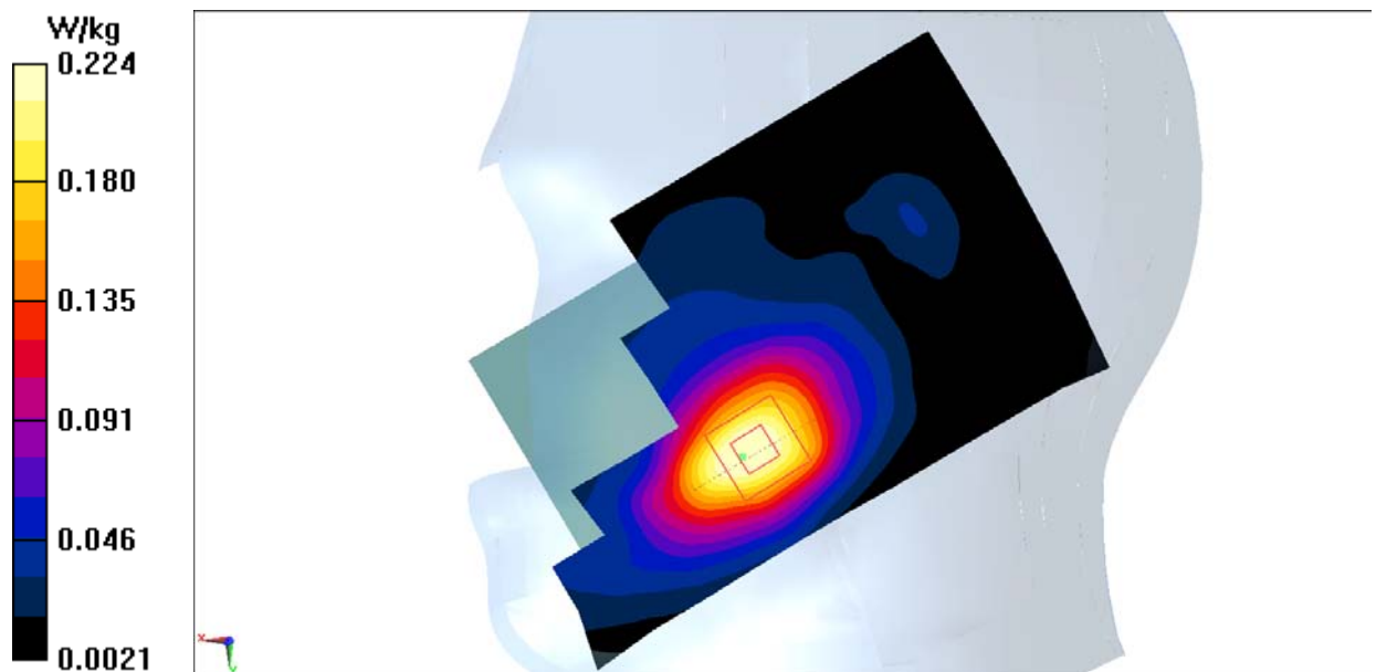
Fig.11 LTE Band2
