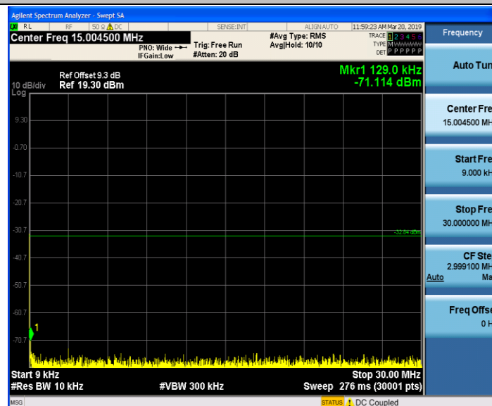
11B_Ant1_2462_0.009~30
