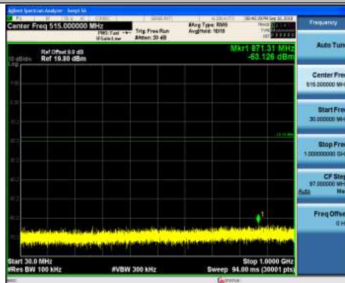
11N20MIMO_Ant1_2457_30~1000
