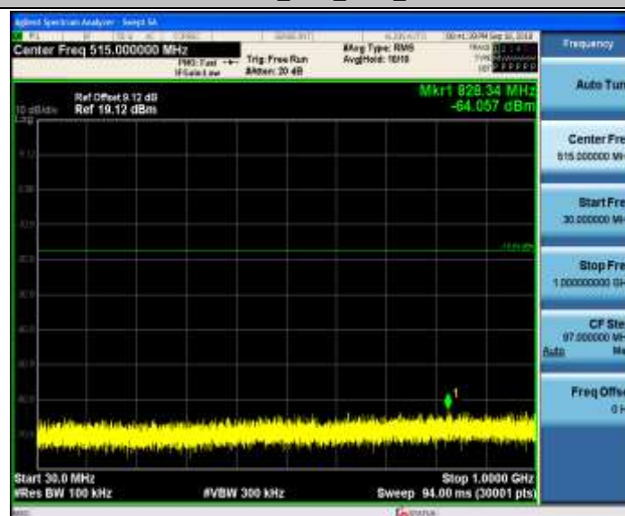
11N20MIMO_Ant2_2417_30~1000
