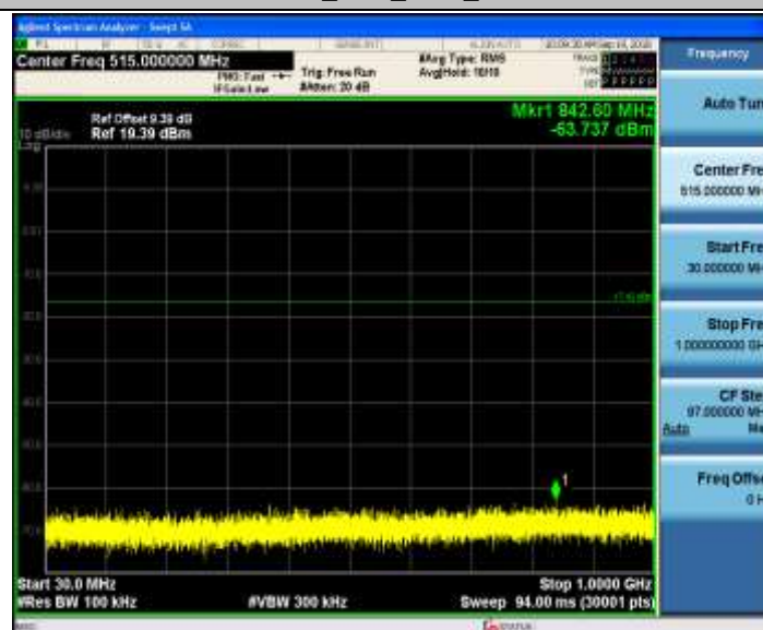
11G-CDD_Ant2_2422_30~1000
