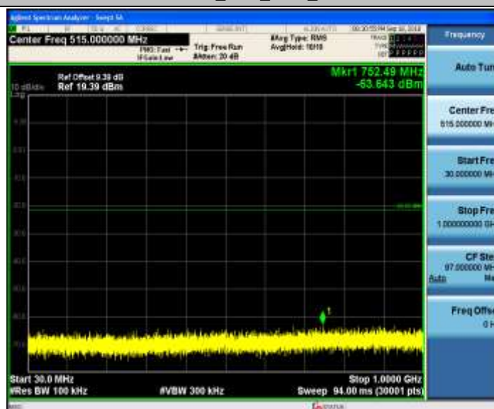
11N40SISO_Ant2_2442_30~1000
