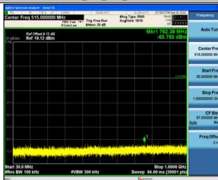
11B_Ant2_2417_30~1000
