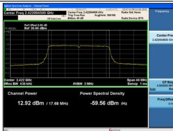
11N20MIMO_Ant2_2422
