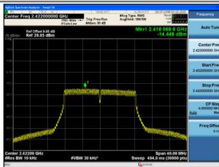
11G_Ant2_2422
