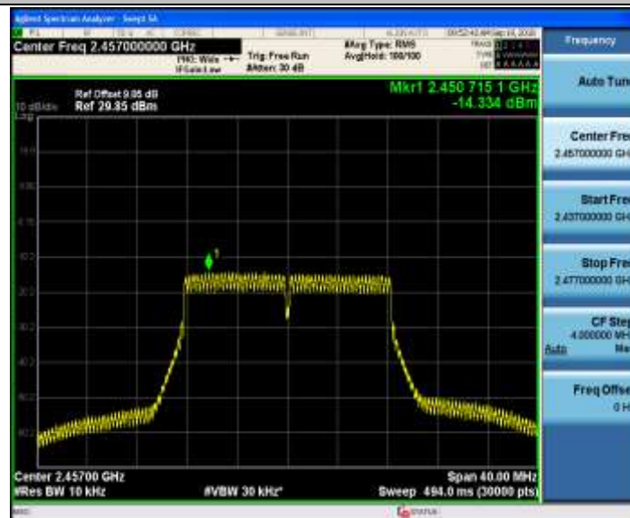
11G-CDD_Ant2_2457
