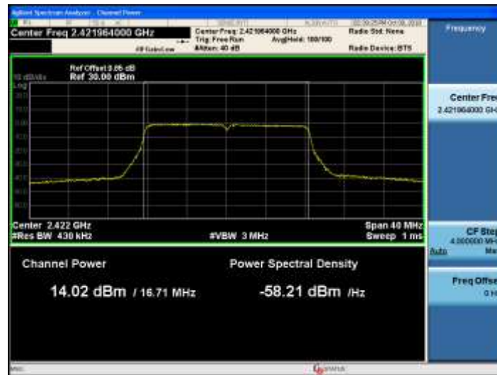
11G_Ant2_2422
