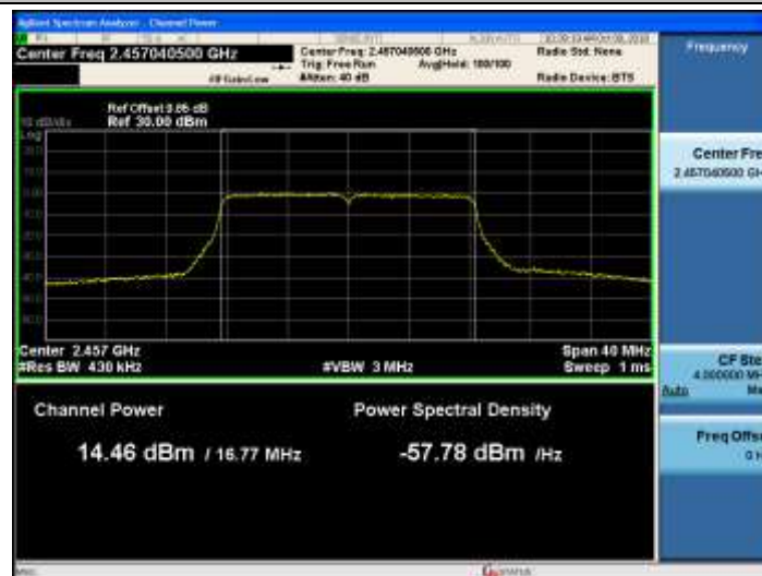
11G_Ant2_2457
