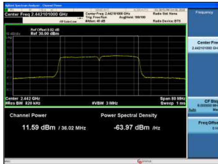
11N40MIMO_Ant2_2442
