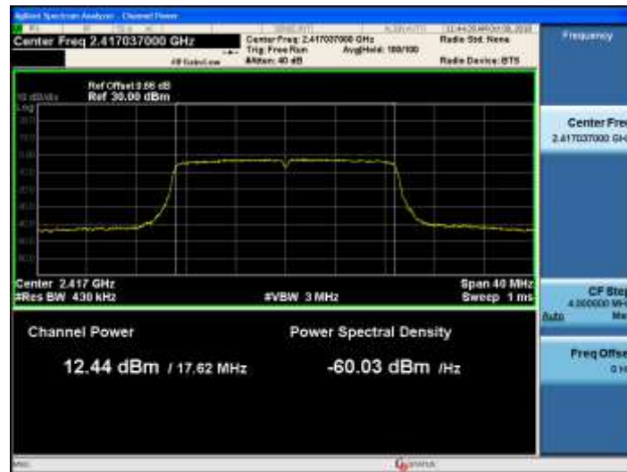
11N20MIMO_Ant2_2417
