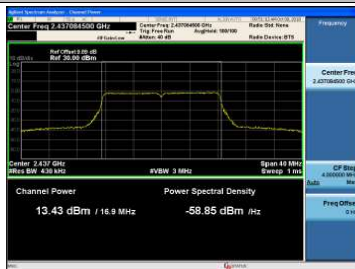
11G_Ant2_2437
