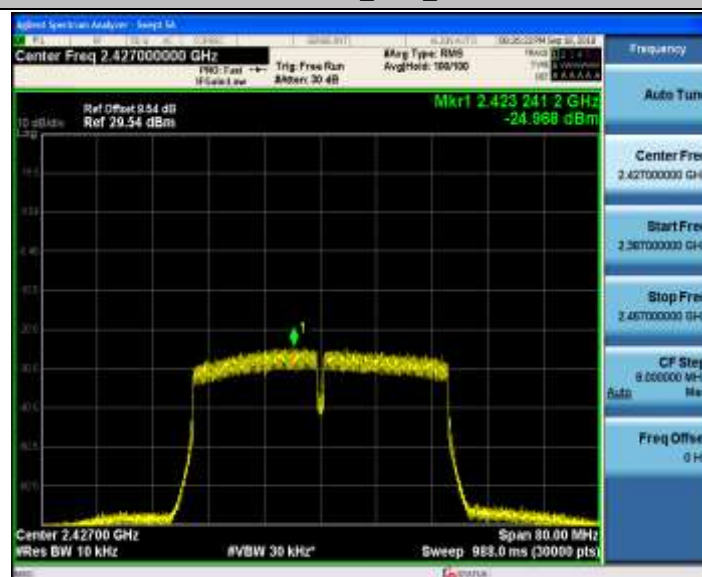
11N40SISO_Ant2_2427
