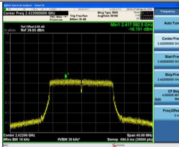
11N20SISO_Ant2_2422
