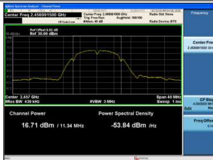
11B_Ant2_2457
