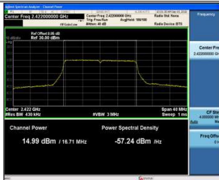
11G-CDD_Ant2_2422
