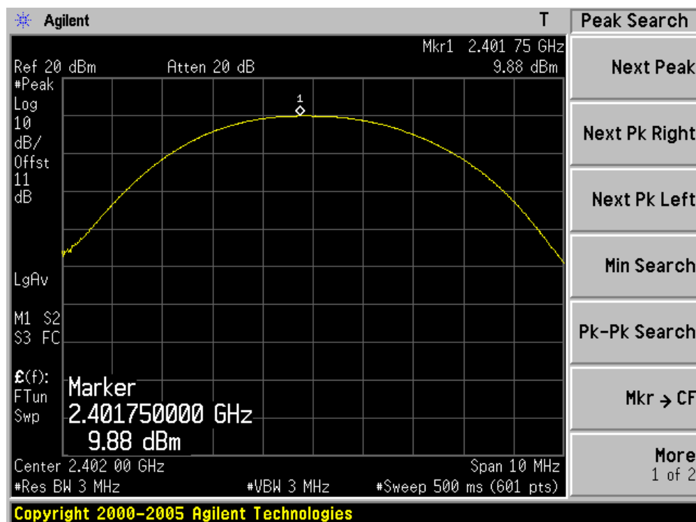
2DH5 2402MHz
